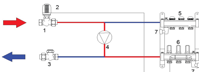
Принципова схема
